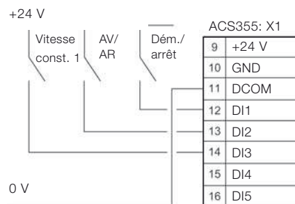
Configuration des entrées logiques (DI) Raccordement PNP avec alimentation externe
