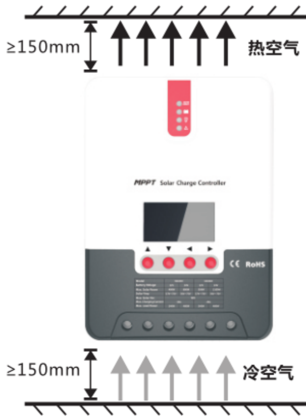
图2.1 安装和散热
